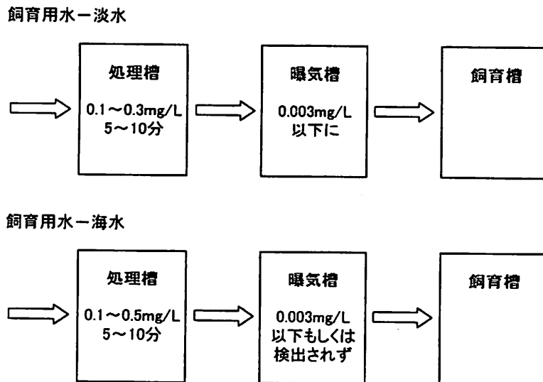
図1. 飼育用水（淡水および海水）のオゾン処理図式
